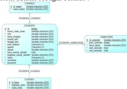
Gambar 10. ERD Sistem
